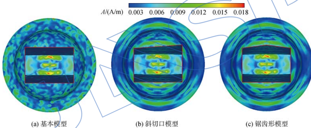
图 10 水平极化方式下 0^\circ 入射方位角时的腔体感应电流线密度分布
