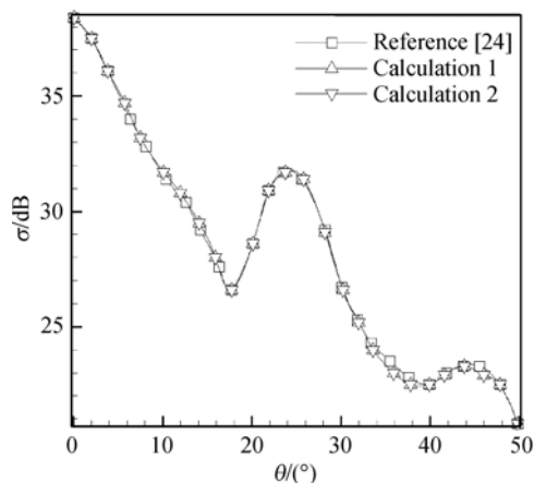
图7 垂直极化下 RCS 分布对比
