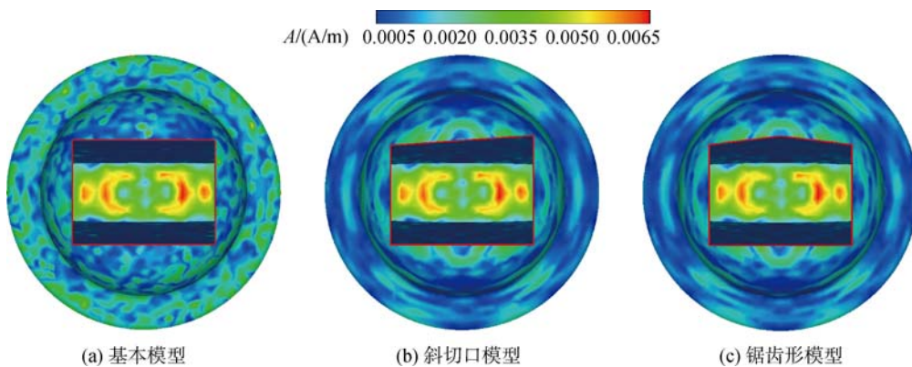
图 11 垂直极化方式下 0^\circ 入射方位角时的腔体感应电流线密度分布
