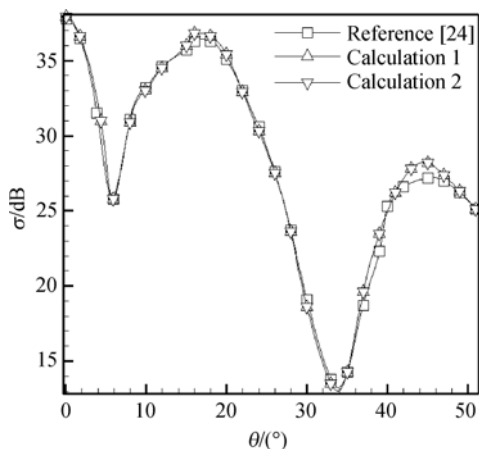
图6 水平极化下 RCS 分布对比
